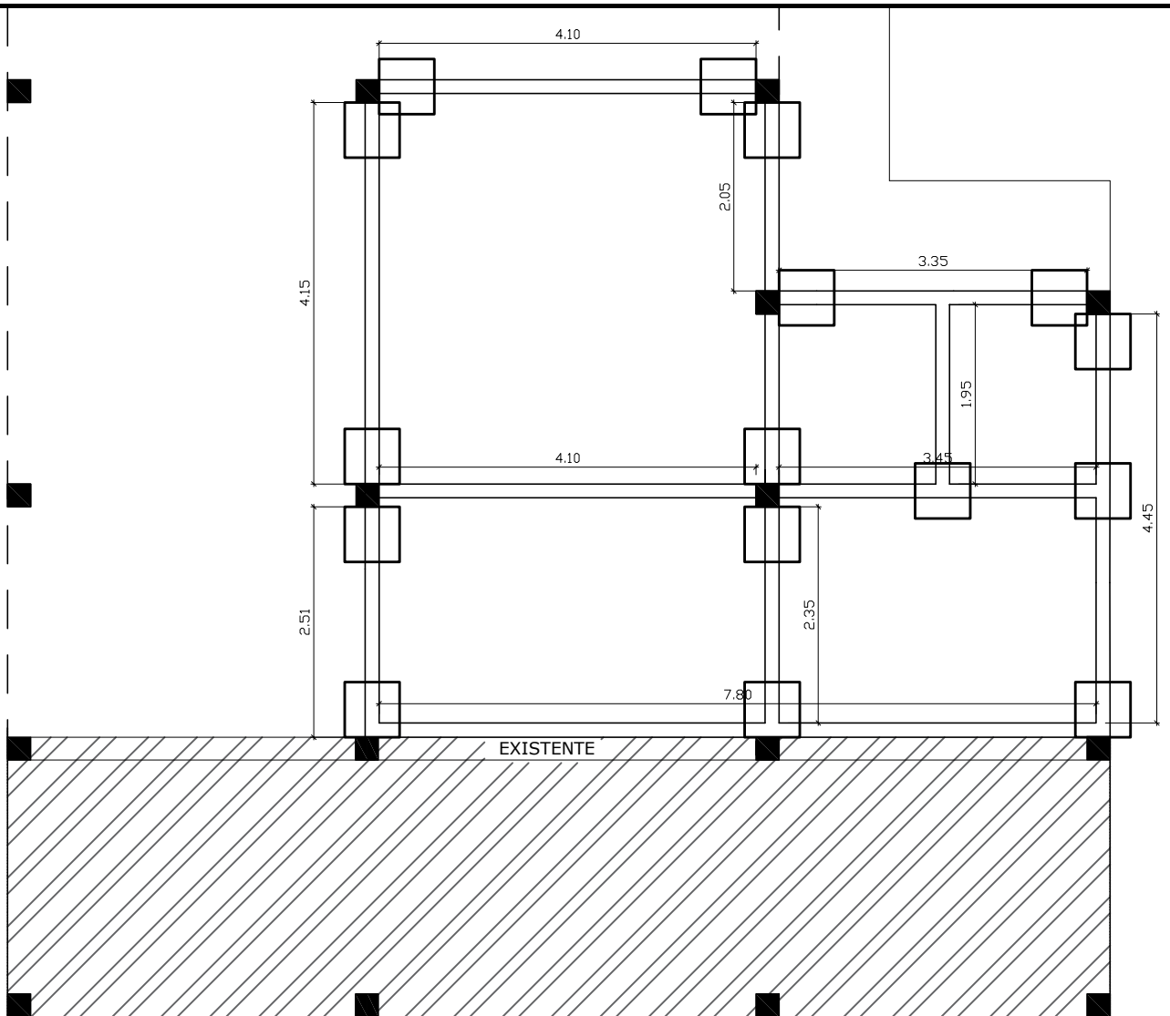
BLOCOS DE FUNDAÇÃO E VIGAS DE BALDRAME
